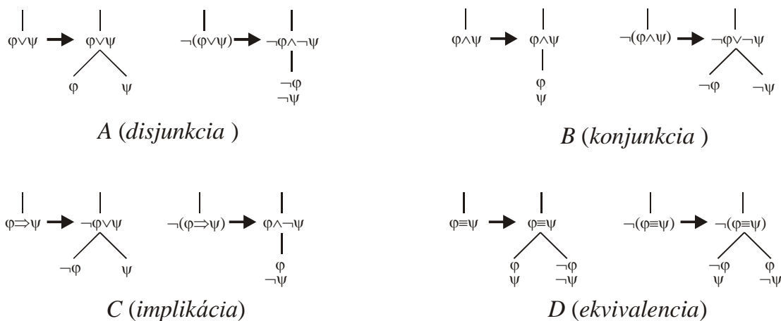
Obrázok 5.1. Základné módy tvorby binárneho stromu v metóde sématických tabiel. (A) Rozklad disjunkcie a jej negácie, (B) rozklad konjunkcie a jej negácie, (C) rozklad implikácie a jej negácie a (D) rozklad ekvivalencie a jej negácie.
